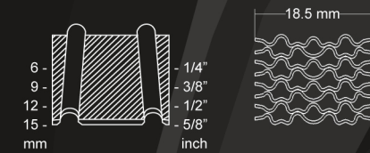
CF185S
