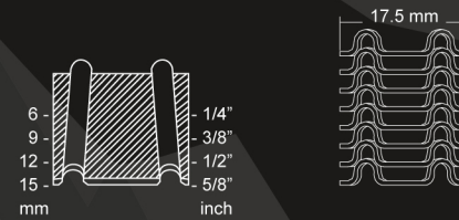
CF175P
